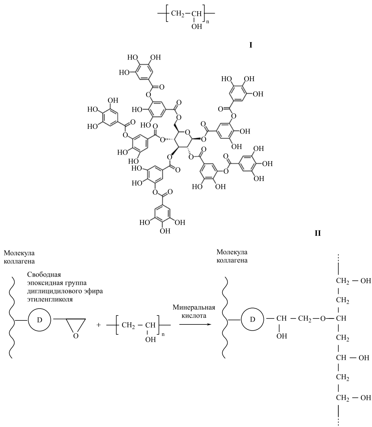
Рис. 4. Взаимодействие эпоксидных групп ДЭЭ-стабилизированного ксеноперикарда с гидроксильными группами поливинилового спирта
