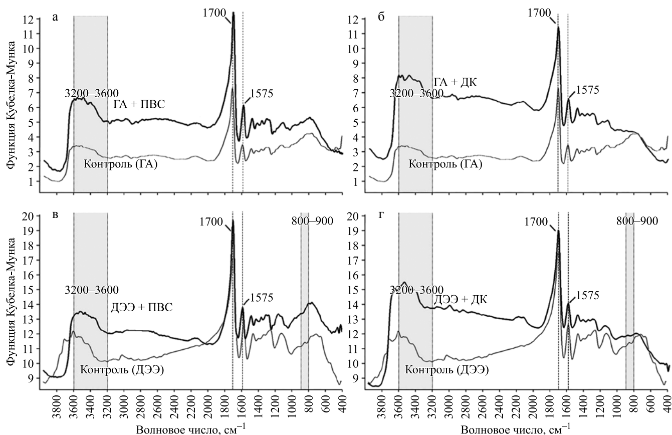
Рис. 1. ИК-спектры диффузного отражения биологического материала, консервированного ДЭЭ и ГА и модифицированного ПВС и ДК: а – сравнение спектров ГА-перикарда, обработанного ПВС, с контролем; б – сравнение спектров ГА-перикарда, обработанного ДК, с контролем; в – сравнение спектров ДЭЭ-перикарда, обработанного ПВС, с контролем; г – сравнение спектров ДЭЭ-перикарда, обработанного ДК, с контролем
