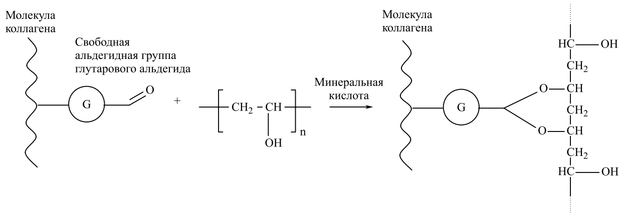
Рис. 5. Образование полуацеталей в результате взаимодействия альдегидной группы глутарового альдегида и двух ближайших гидроксильных групп поливинилового спирта
